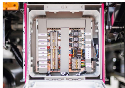
Central elbox som gör det enkelt att diagnostisera och underhålla systemen.
